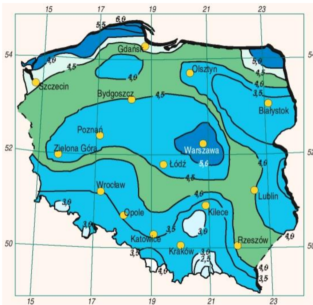
Rycina 18. Średnioroczna prędkość wiatru (m/s) na wysokości ponad 30 m nad powierzchnią ziemi w terenie z przeszkodami do 3 m
